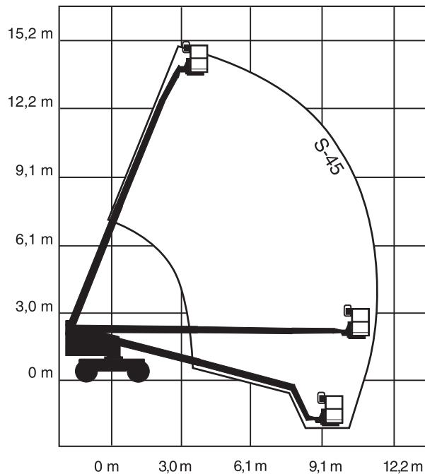
S-45 Liikealuekaavio
