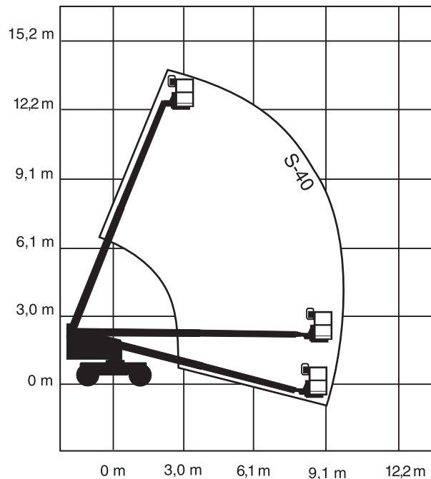
S-40 Liikealuekaavio
