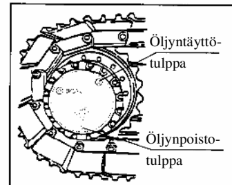
Vaihdelaatikko (vaihdeöljy)
